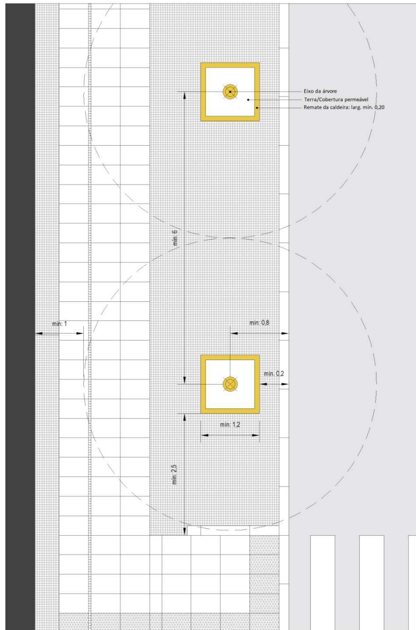
Figura 1 – Implantação de caldeiras em circuito pedonal
