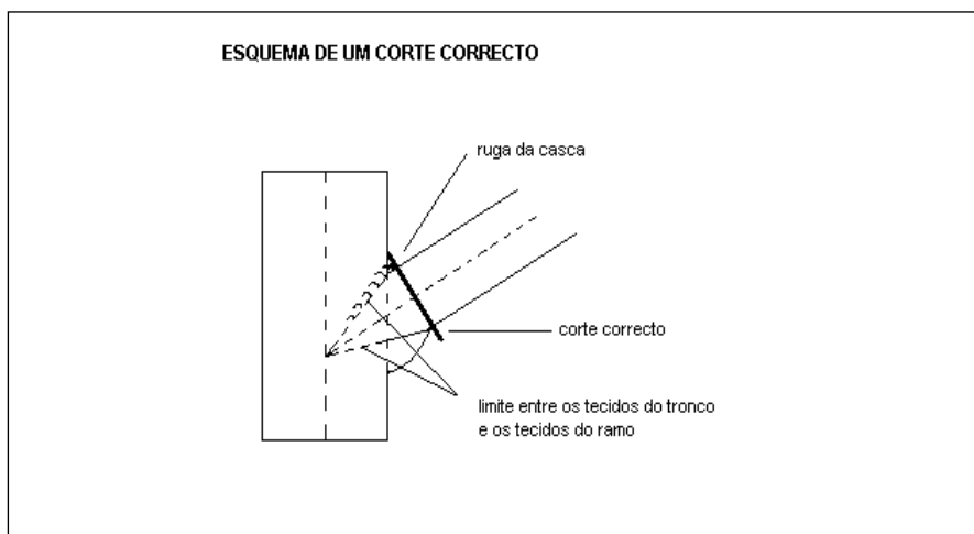
Figura A.1.2 - Esquema de corte correto.
